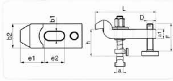
Ayarlanabilir Destek Civatalı Kombine Bağlama Z Pabuç
